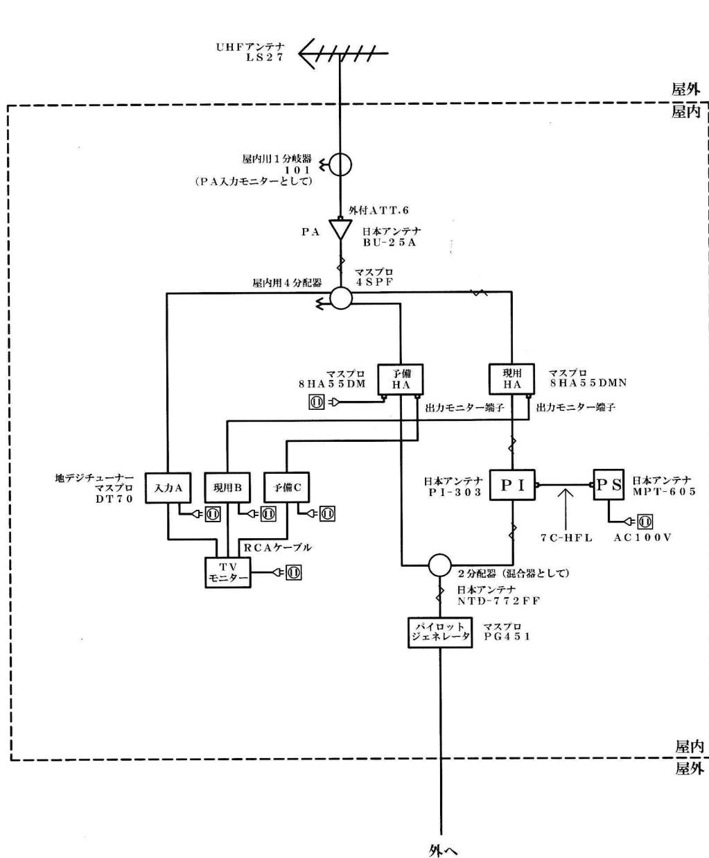
配線系統図
