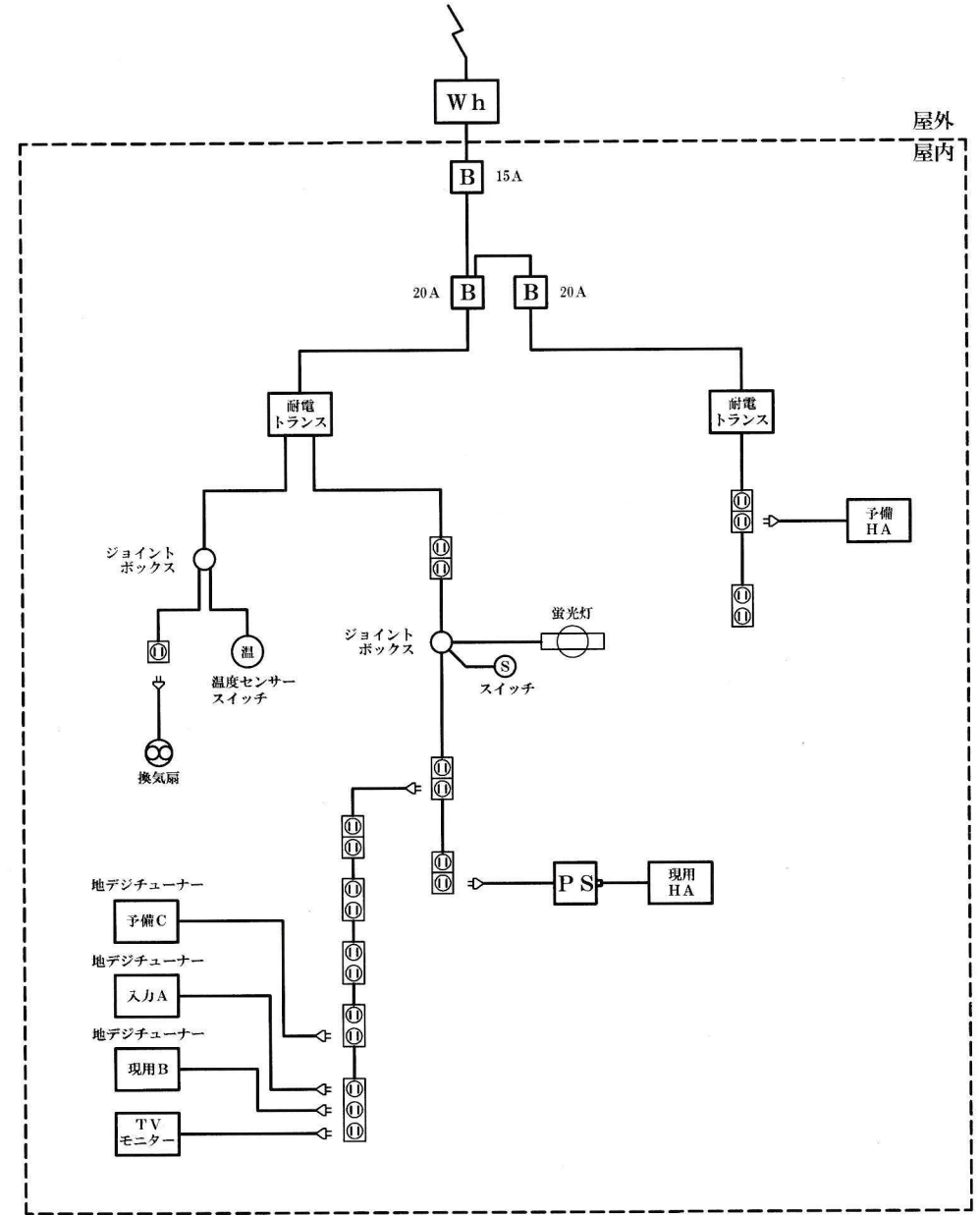
電源系統図
